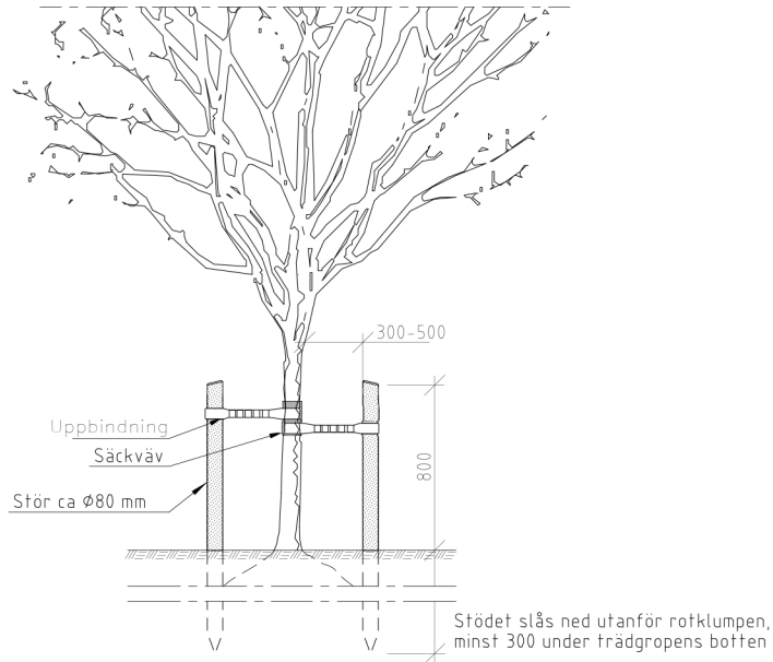
SEKTION Skala 1:20
