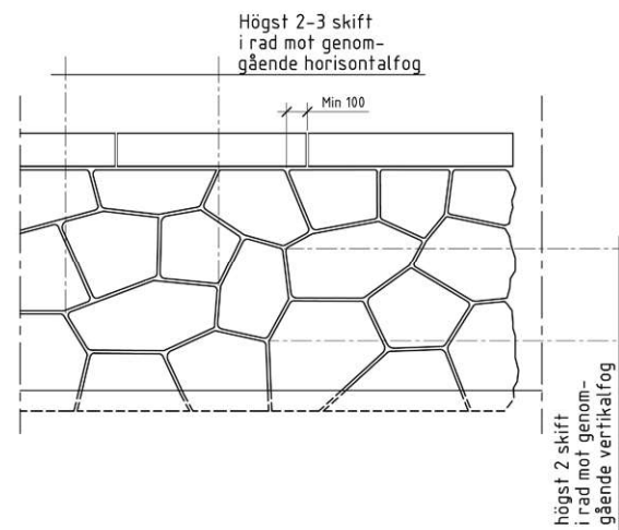
FASAD Skala 1:20
