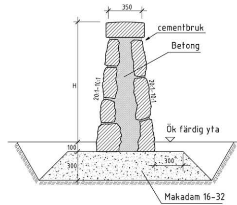
SEKTION Skala 1:20
